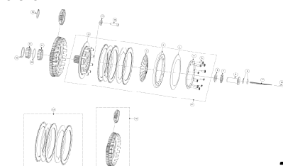
EMBRAGUE CLUTCH
