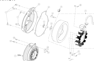
ENCENDIDO IGNITION
