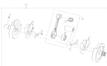
CIGUEÑAL CRANKSHAFT
