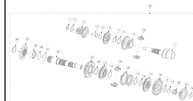
ENGRANAJES CAMBIO GEAR SET
